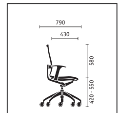
open up met rugleuning met membraan- bespanning, neksteun, vlak kussen, aluminiumvoet gepolijst
