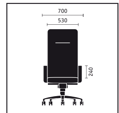
Directiebureaustoel met hoge rugleuning met geïntegreerde neksteun met "independent fit"- technologie.
